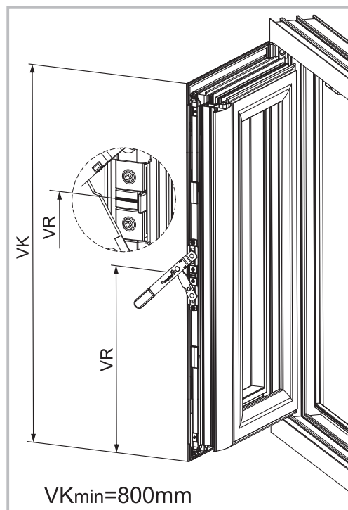
Bravica pomoćnog krila u zatvorenom položaju Вспомогательный замок створки в закрытом положении Lock for double sash in closed position
