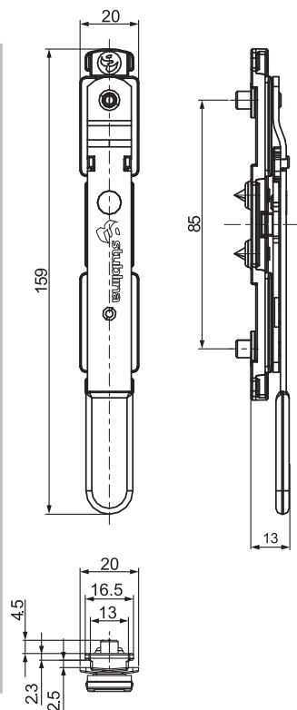
Bravica pomoćnog krila u zatvorenom položaju Вспомогательный замок створки в закрытом положении Lock for double sash in closed position
